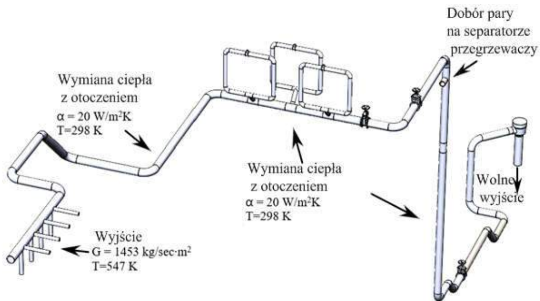
Fig. 1. Schemat obliczeniowy.
