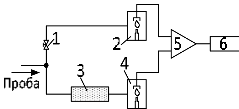
Рисунок 1. Диференційна схема вимірювання вуглеводнів за вирахуванням метану.
