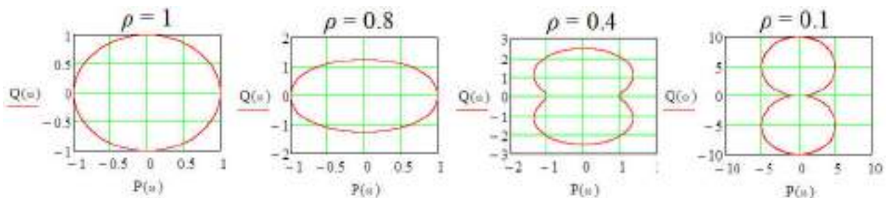
Рисунок 2 – АФХ бурильної колони при зміні ступеню узгодженості
