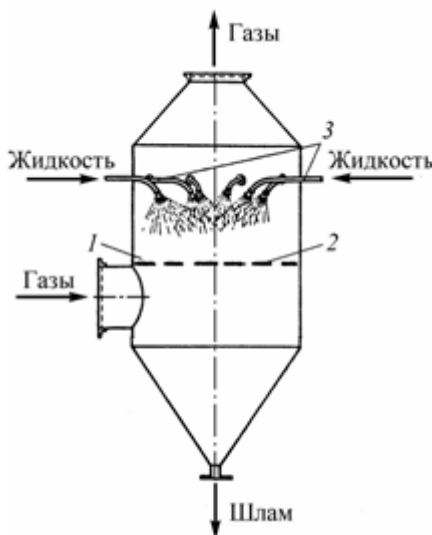
1 – корпус; 2 – газорозподільна решітка; 3 – форсунки Рисунок 4.1 – Порожнистий форсунковий скрублер
