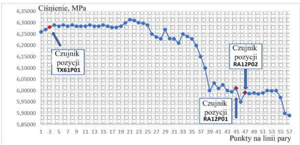
Rysunek 3. Spadek ciśnienia w przewodzie pary nr 2 z wytwornicy pary nr 2.
